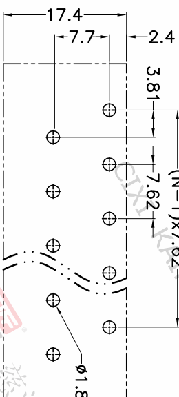
P.C.B.LAYOUT
